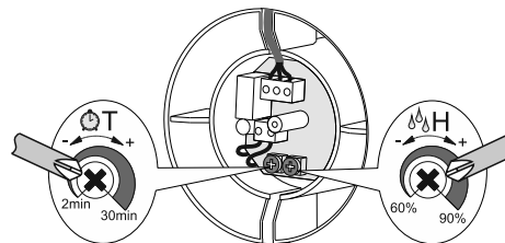
серия СИЛЕНТА-СТ, СИЛЕНТА-СТН
