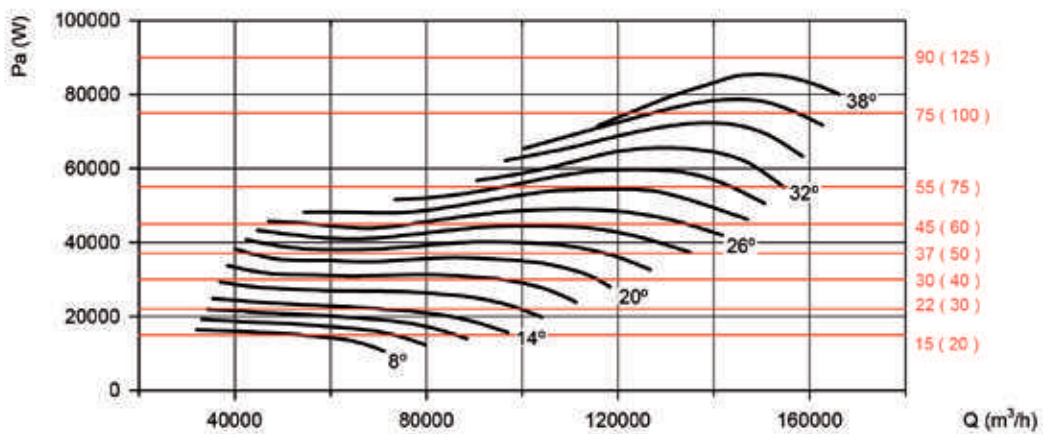
Potencia absorbida
