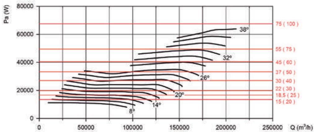
Potencia absorbida
