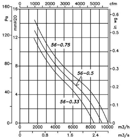
6 Polos=1000 r/min
