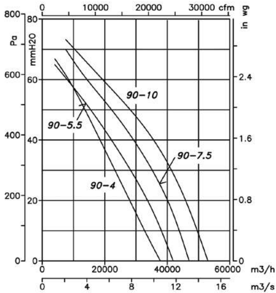
4 Polos=1500 r/min
