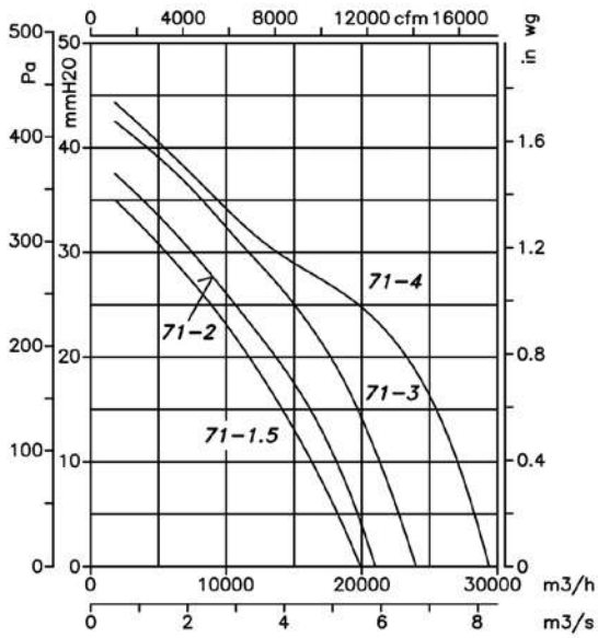
4 Polos=1500 r/min
