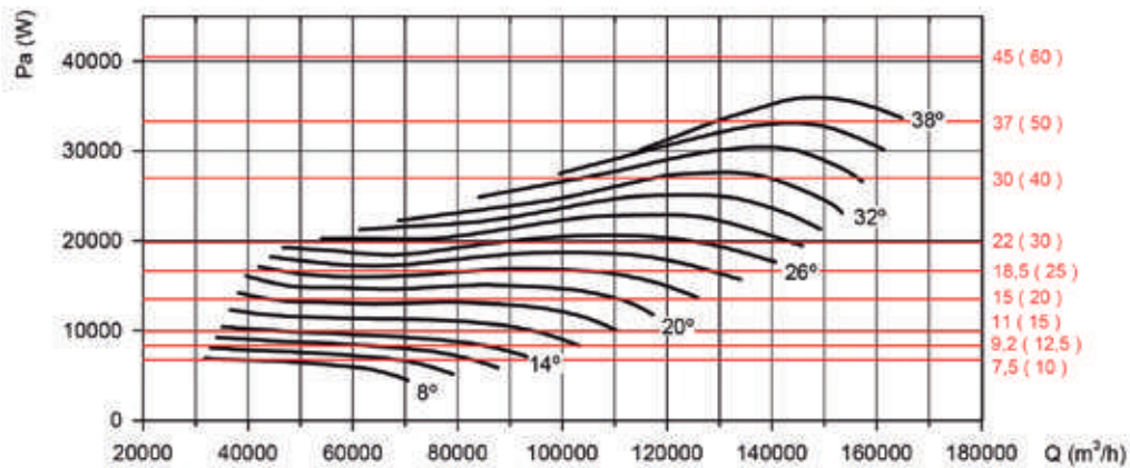
Potencia absorbida
