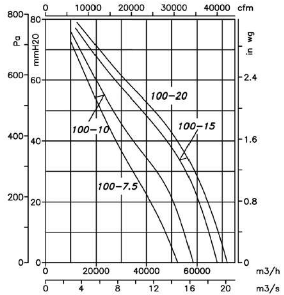
4 Polos=1500 r/min
