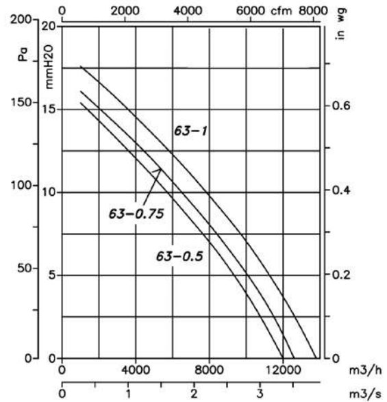
6 Polos=1000 r/min
